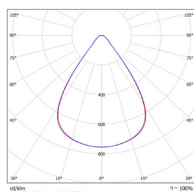
D75 Faisceau 75°
