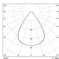
D75 Faisceau 75°
