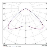
D120 Faisceau 120°
