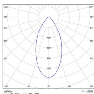
D60 Faisceau 60°
