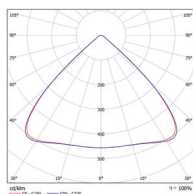
D90 Faisceau 90°
